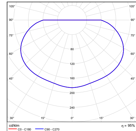
Lichtaustritt 1 / Polare LVK
